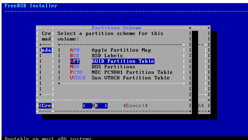
Abbildung 2.17. Partitionen manuell anlegen
